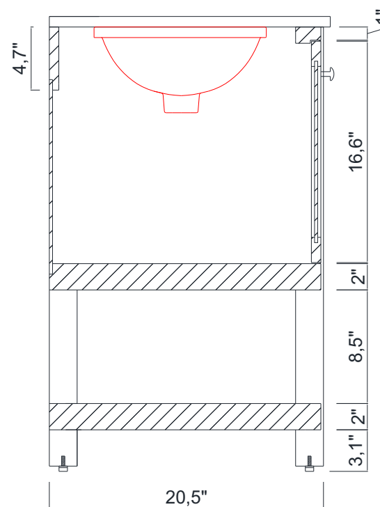
A-A SECTION
